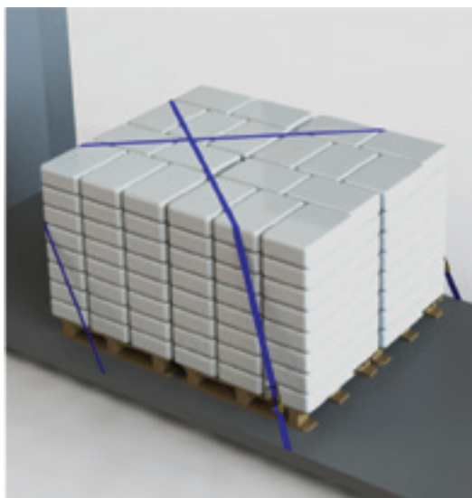
Figura 73: quattro pallet con ancoraggio antirimbalo incrociato
