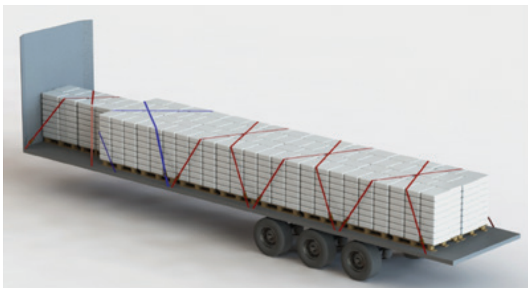
Figura 74: rimorchio con una combinazione di bloccaggio e ancoraggio per attrito e antirimbalo incrociato
