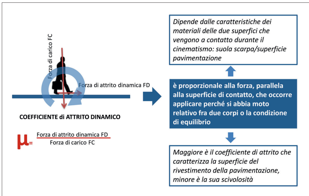
Figura 2: Calcolo del coefficiente di attrito dinamico
